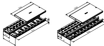
FS-FT38 (2 or 3 compartments) FS-FT38 (2 oder 3 Kompartimente)
